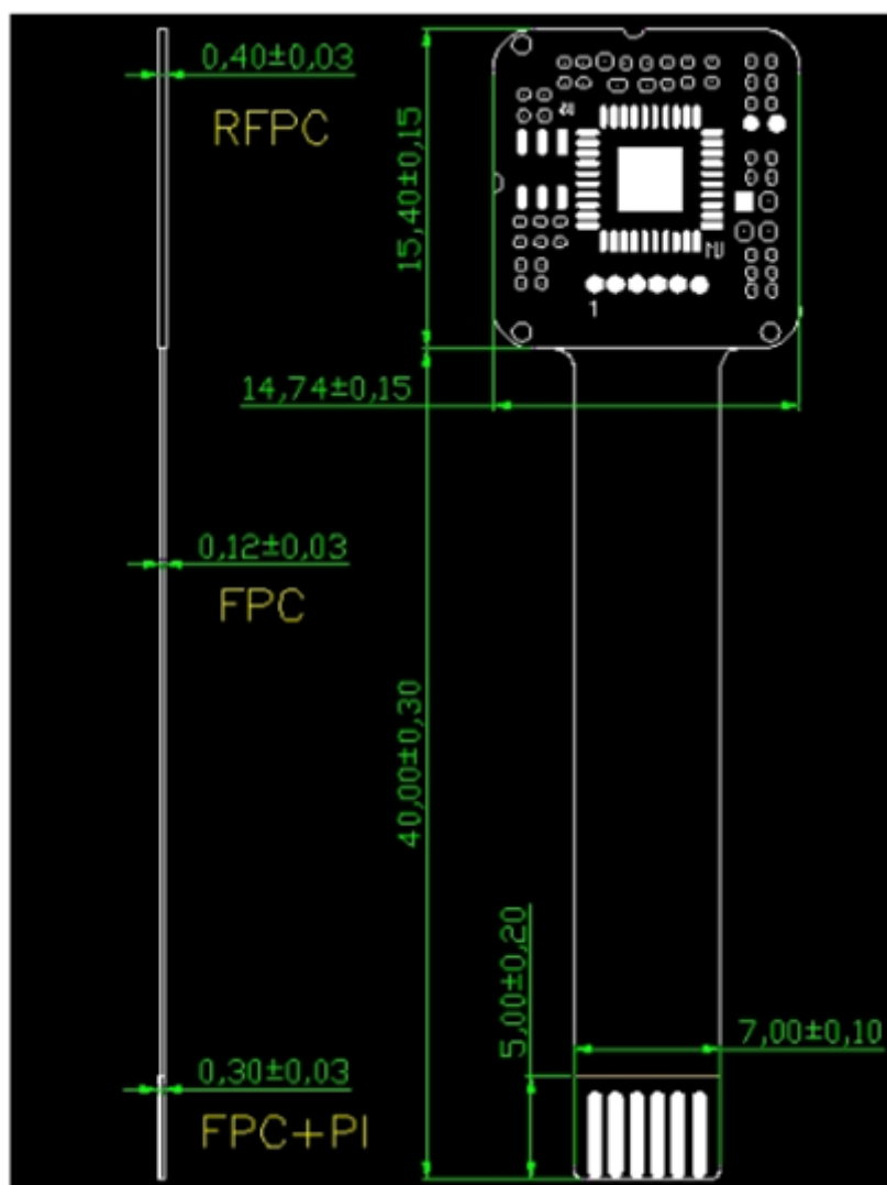
FPC 结构尺寸
