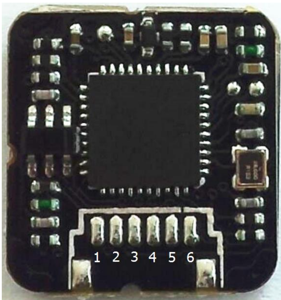
图 5.3.1 管脚说明
